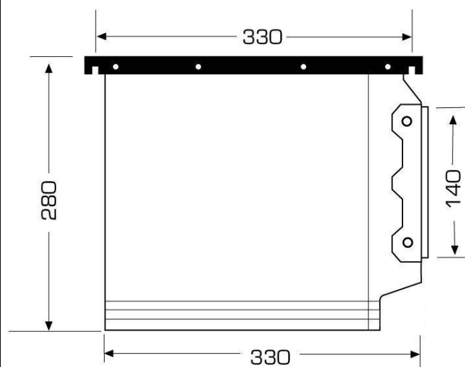
Schema Prodotto
